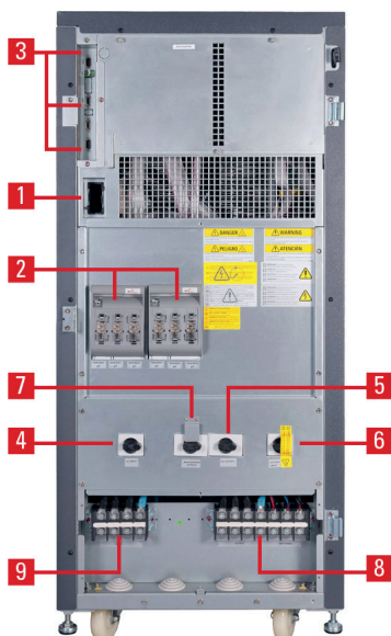
SLC-7,5-200-CUBE3+
